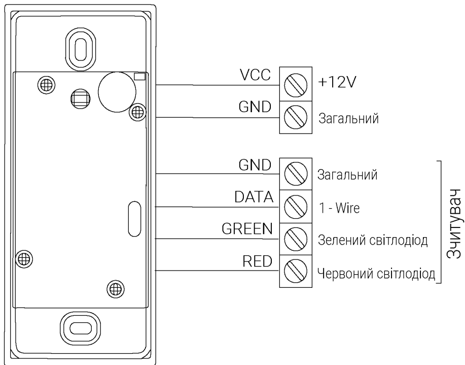
Рисунок 1 - Підключення по інтерфейсу 1-Wire
