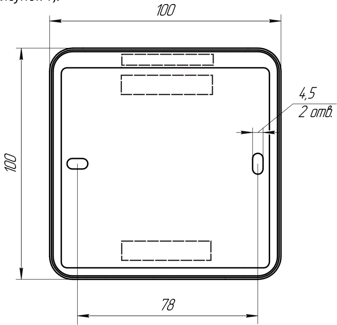
Рисунок 1 – Розмітка отворів на основі корпуса модуля
