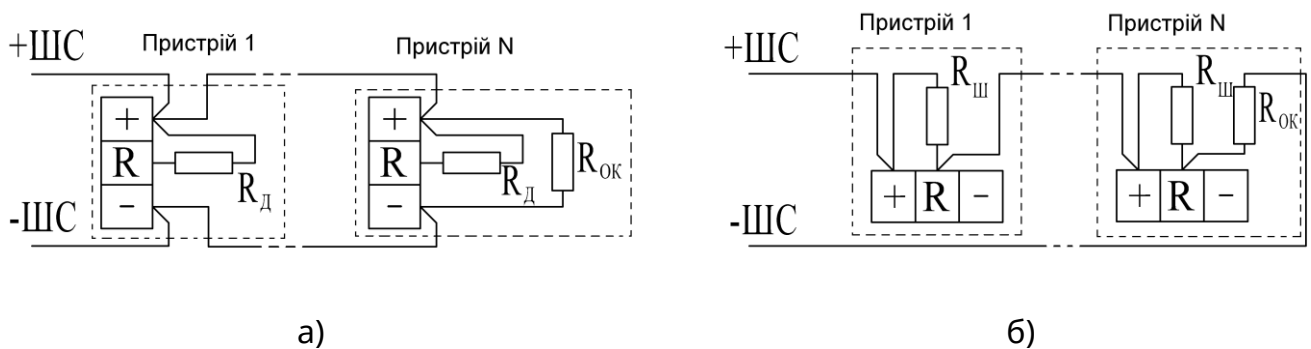
Рисунок 2 - Схема підключення пристроїв:
