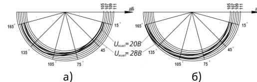
Рисунок 2 – Акустичні діаграми ОСЗ «Джміль-2» (24V):
