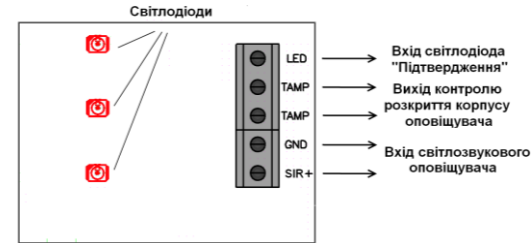
Рисунок 4 - Схема підключення оповіщувача
