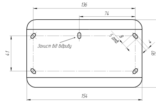
Рисунок 3 – Розмітка отворів на основі корпусу оповіщувача
