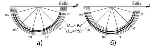
Рисунок 1 – Акустичні діаграми ОСЗ «Джміль-2»: а) –робоче положення, б) – повернене на 90° за годинниковою стрілкою положення
