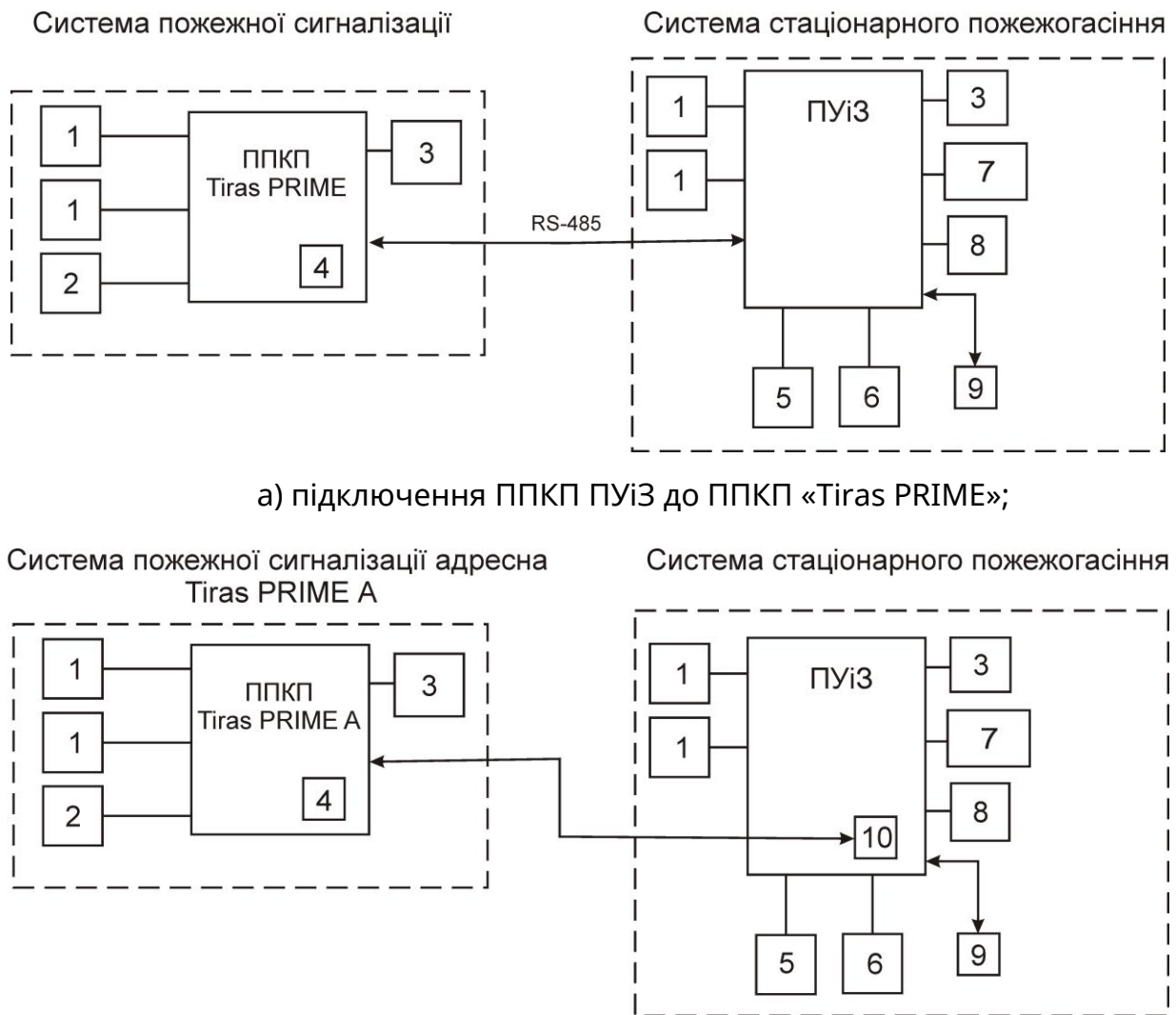
б) підключення ППКП ПУІЗ до ППКП «Tiras PRIME A».
