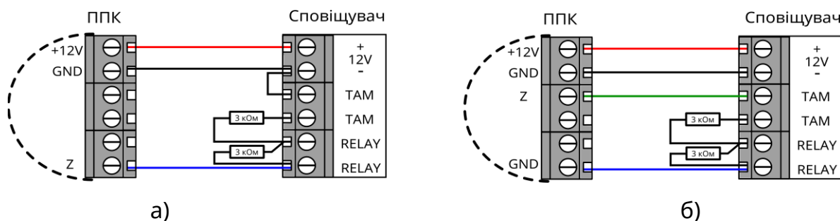
Рисунок 2.6 – Приклади підключення сповіщувачів по типу 2EOL
