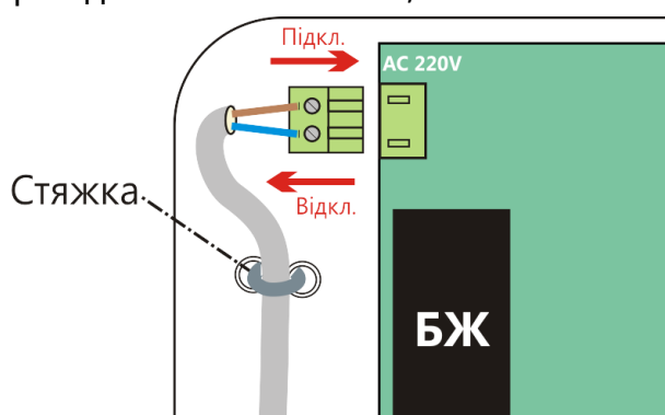
Рисунок 2.4 – Підключення роз'єму 220 В
