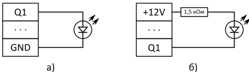
Рисунок 2.8 – Схеми підключення індикаторів підтвердження
