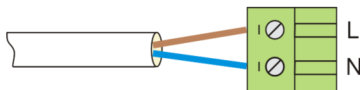
Рисунок 2.3 – Підключення кабелю до роз'єму
