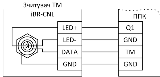
Рисунок 2.9 – Схема підключення зчитувача ключів TM
