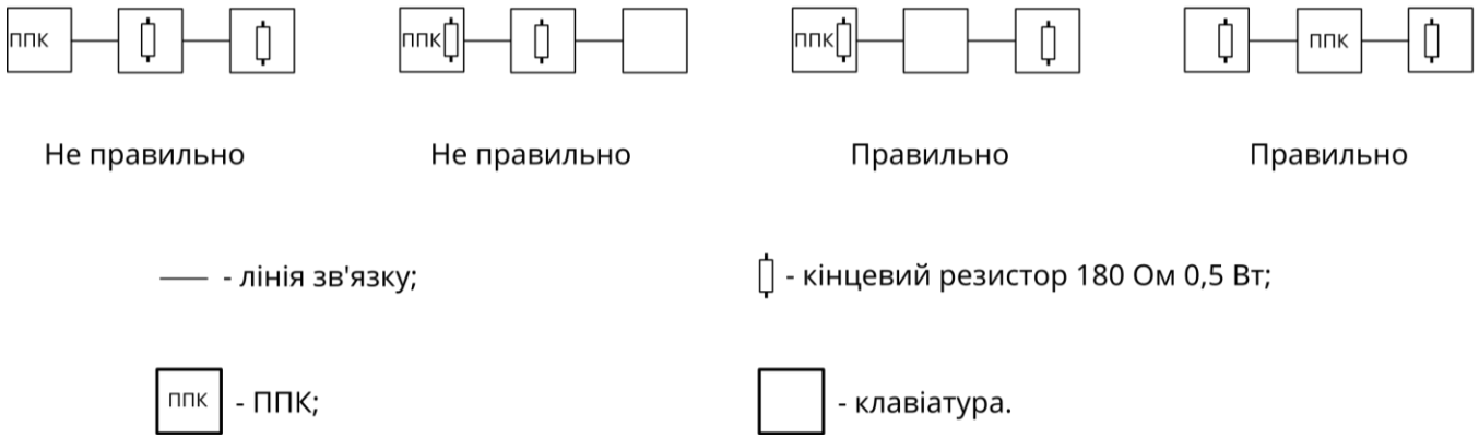
Рисунок 2.1 – Варіанти топології шини RS-485
