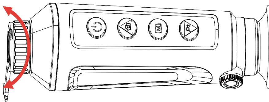
Рисунок 3-2 Регулювання фокуса
