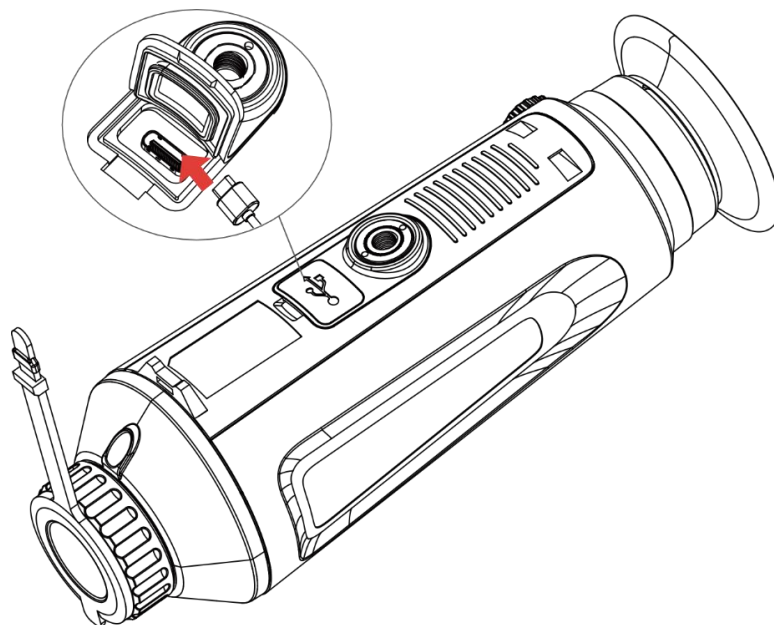
Рисунок 2-1 Підключення кабелю
