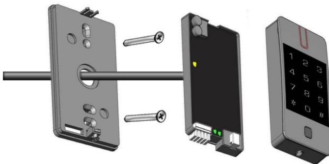
Рис 13. Установка контроллера
