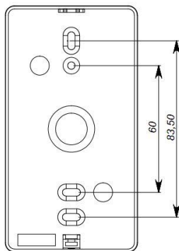
Рис 12. Задняя
