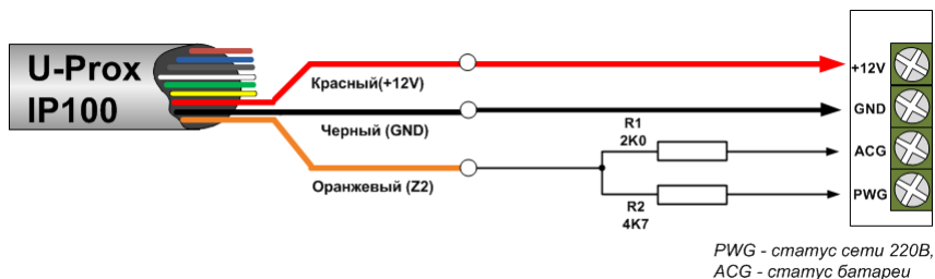
Рис.18. Подключение шлейфа контроля 220В и АКБ к PSU
