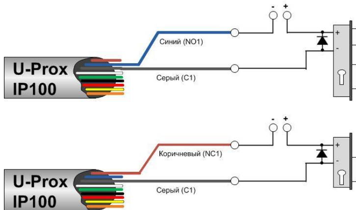
Рис.19. Подключение замков
