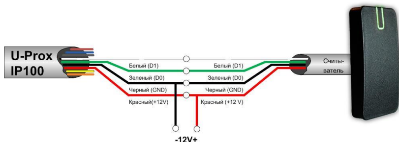
Рис. 14. Подключение внешнего считывателя
