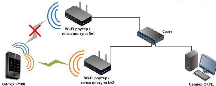
Рис 6. Работа с несколькими Wi-Fi точками доступа
