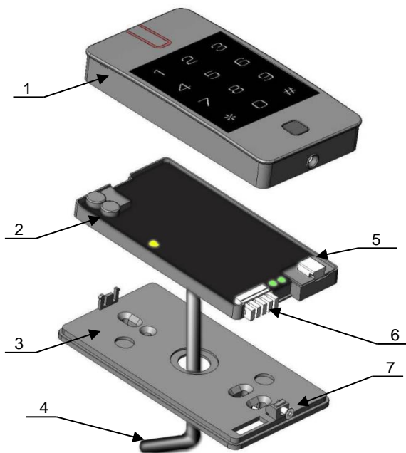
Рис. 2. Внешний вид компонентов U-Prox IP100
