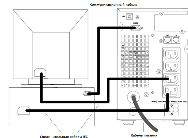
Рис. 3. Пример подключения устройств Plug&Play
