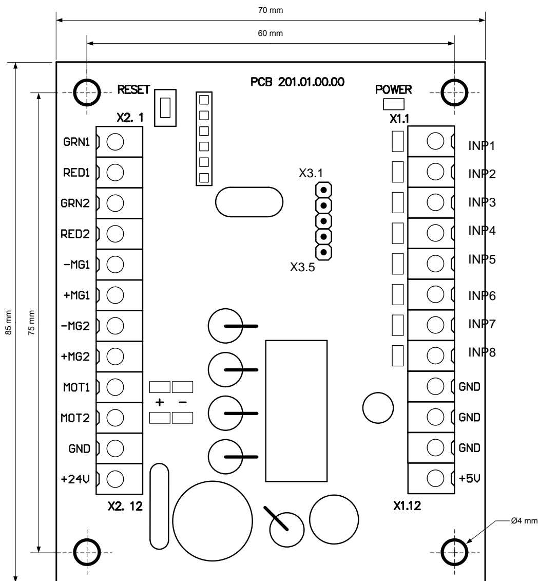
Рисунок 3 – Внешний вид контроллера РСВ.201.01.00.00
