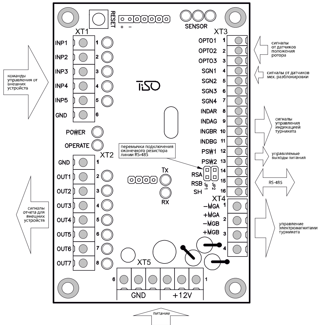
Рисунок 2 – Внешний вид контроллера PCB.112.21.20.00
