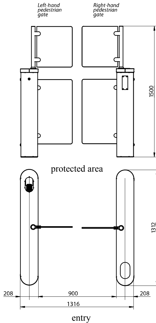
Figure 1 – «SWEEPER-1» type turnstile
