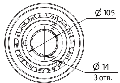
A-A (1:5)
