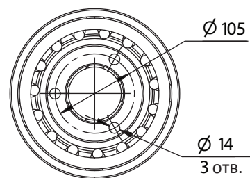
A-A (1:5)
