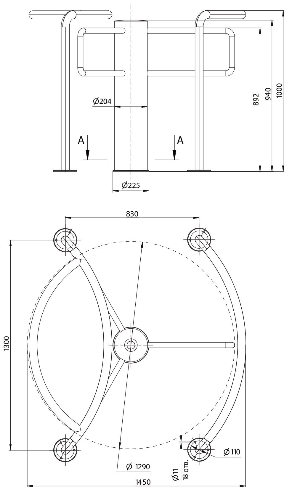
A-A (1:5)
