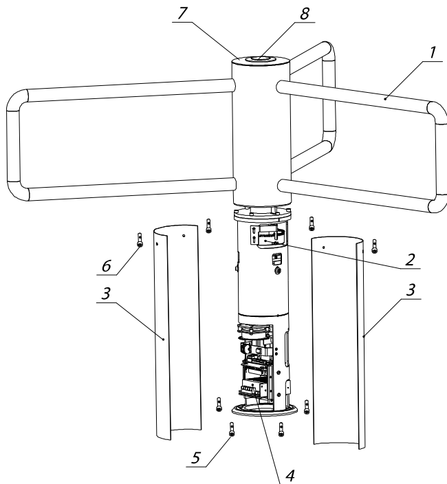
Рисунок 1 – Конструкция роторного турникета ТЗ.РОН.ХС
