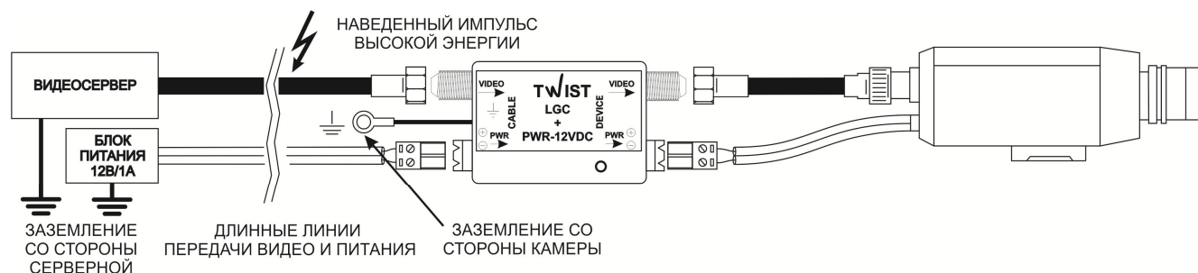
Рис.1 Схема включения TWIST LGC+PWR-12VDC
