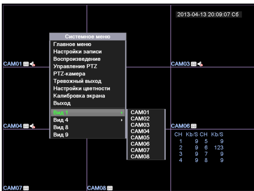
Рис.2.1.1. «Режим live-экрана с открытым всплывающим меню»
