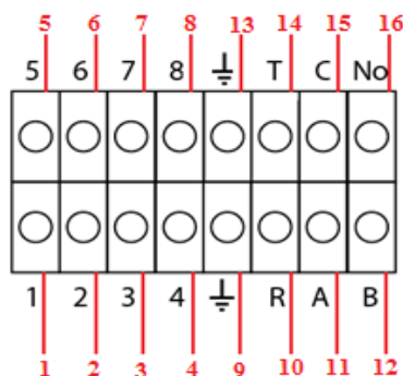
Рис. 1.2.1 «Клеммная колодка регистратора»
