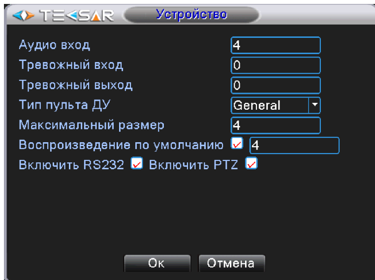
Рис. 4.4.4. Управление. Устройство
