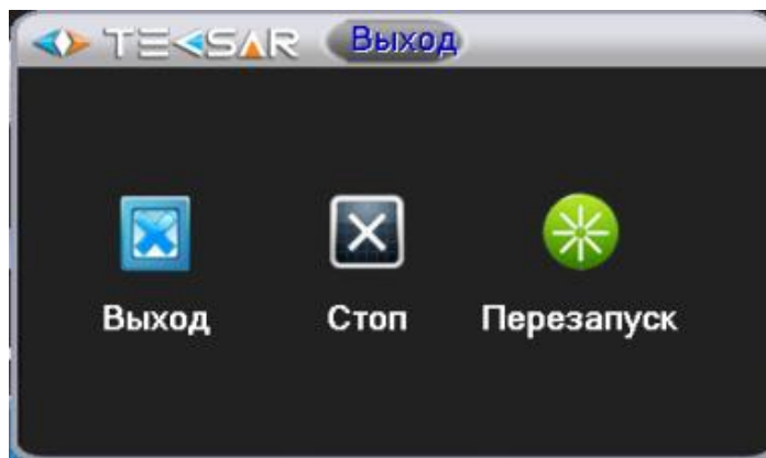
Рис. 3.2.6. «Выход»
