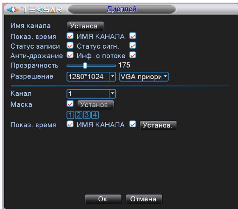
Рис. 4.3.5.1. Настройка. Дисплей
