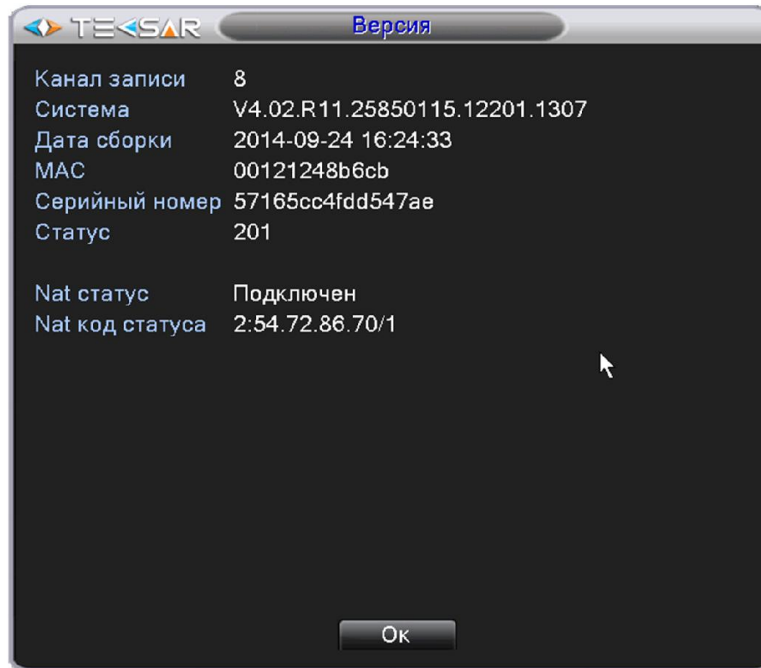
Рис. 4.5.4. Сведения. Версия
