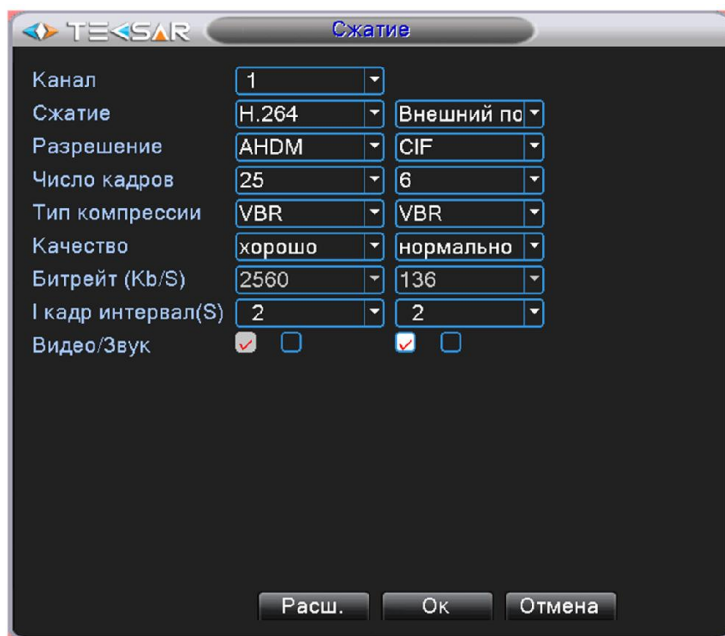
Рис. 4.3.2. Настройка. Сжатие
