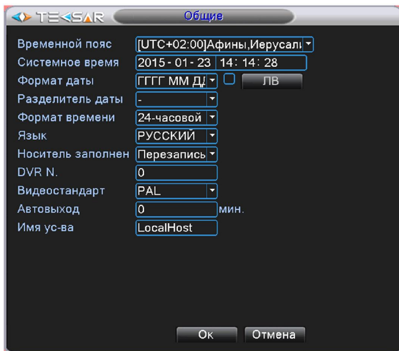
Рис. 4.3.1.1. Настройка. Общие
