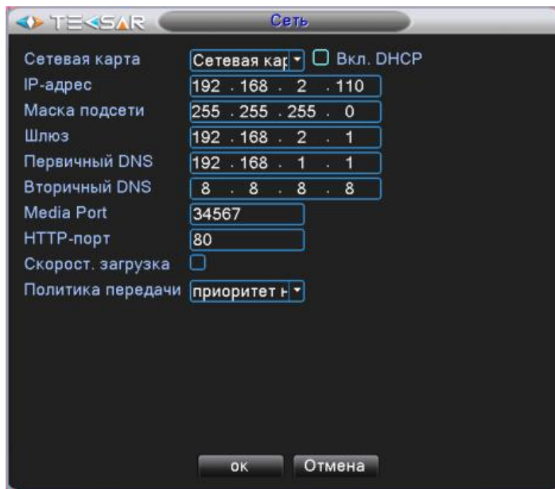
Рис. 4.3.3.1. Настройка. Сеть
