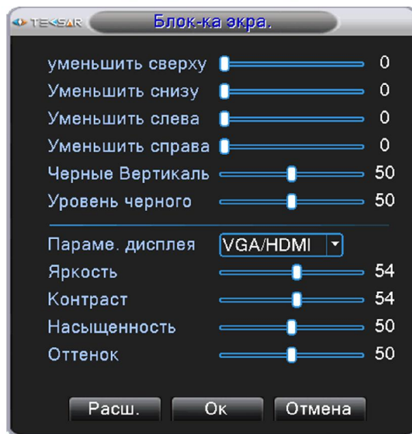
Рис. 3.2.5.1. Блокировка экрана
