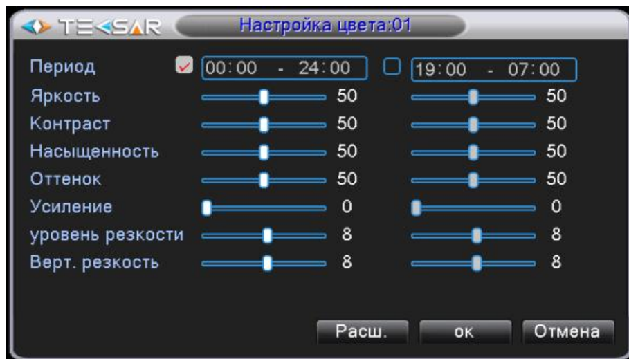
Рис. 3.2.4.1. «Настройки цветности»
