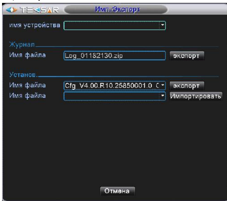
Рис. 4.4.8. Управление. Импорт/экспорт
