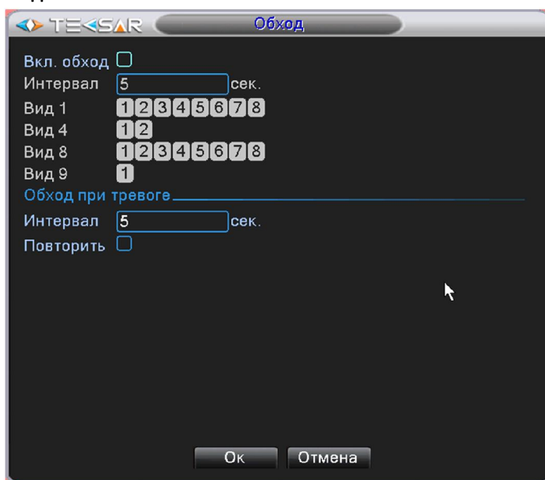
Рис. 4.3.8. Настройка. Обход
