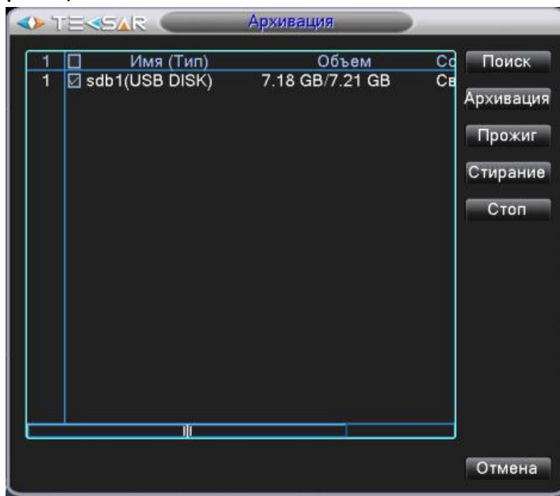
Рис. 4.1.3.1. Запись. Архивация
