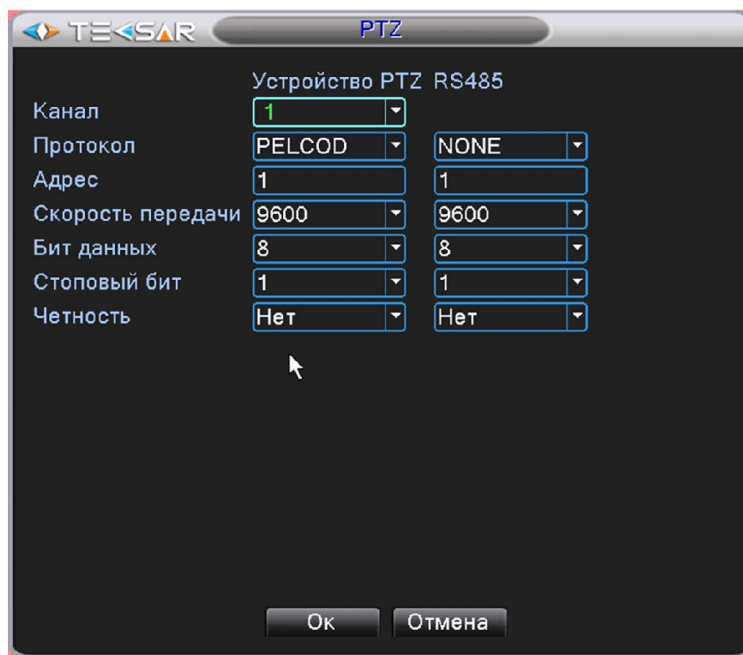
Рис. 4.3.6. Настройка. PTZ
