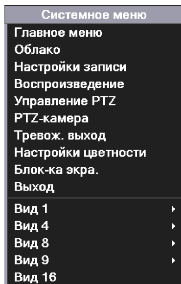
Рис. 3.1. Всплывающее меню
