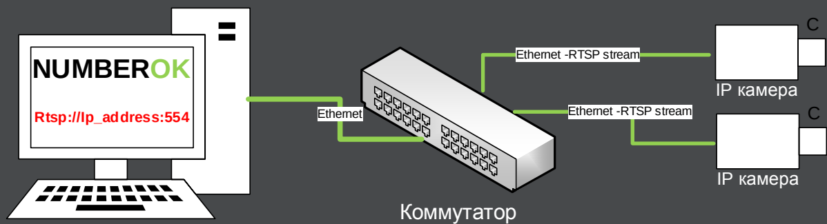
РИСУНОК 4: СХЕМА ПОДКЛЮЧЕНИЯ IP КАМЕР
