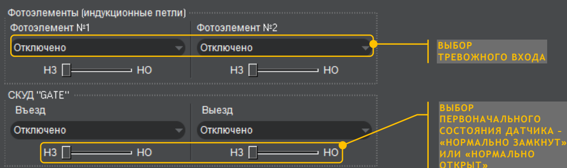
РИСУНОК 49: ПОДКЛЮЧЕНИЕ ТРЕВОЖНЫХ ДАТЧИКОВ
